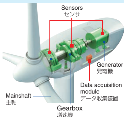
[Wind turbine] 【風力発電装置】
